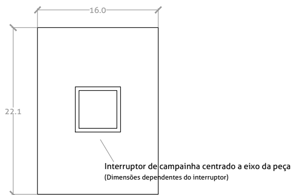
Peça D - topo da caixa Espessura = 0,4 cm
