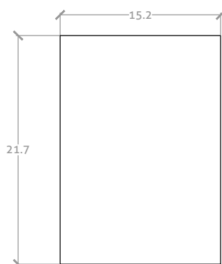
Peça C - fundo da caixa Espessura = 0,7 cm
