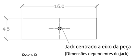
Peça B Espessura = 0,4 cm
